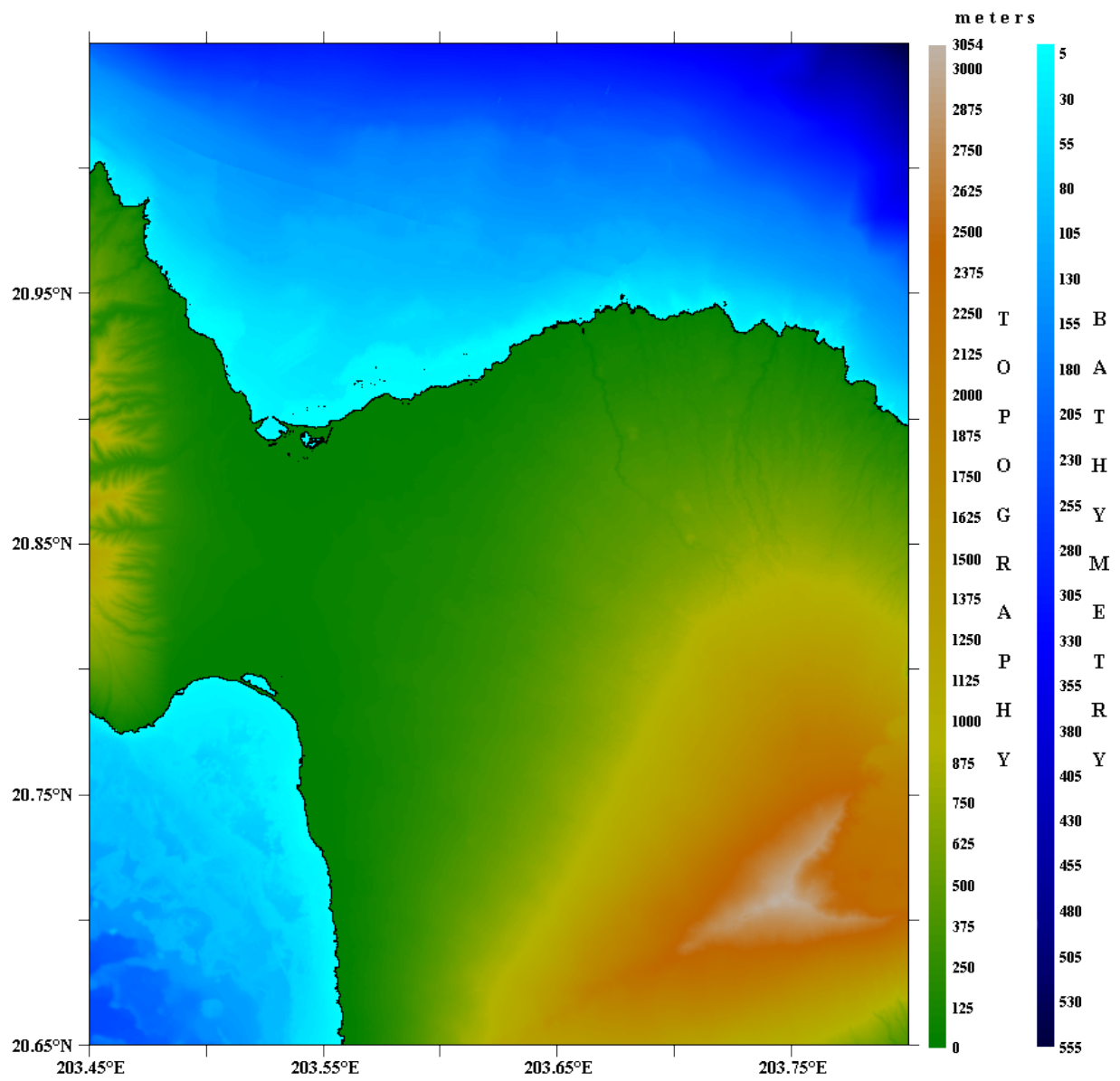
Figure 4. Plot of Kahului DEM.
